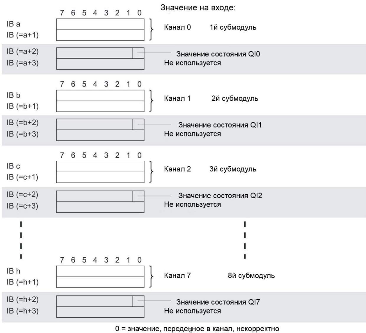
Рисунок 4-3 Пространство адресов модуля для конфигурации 8x1-канальный с оценкой состояния AI 8xU/I HF S QI
