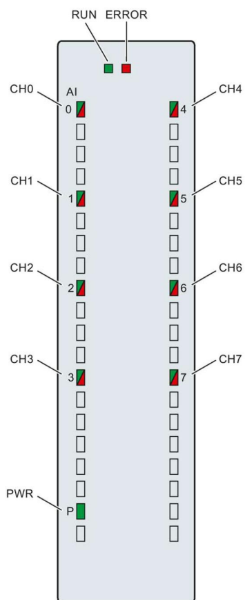
Рисунок 5-1 Светодиодные индикаторы модуля AI 8xU/I HF
