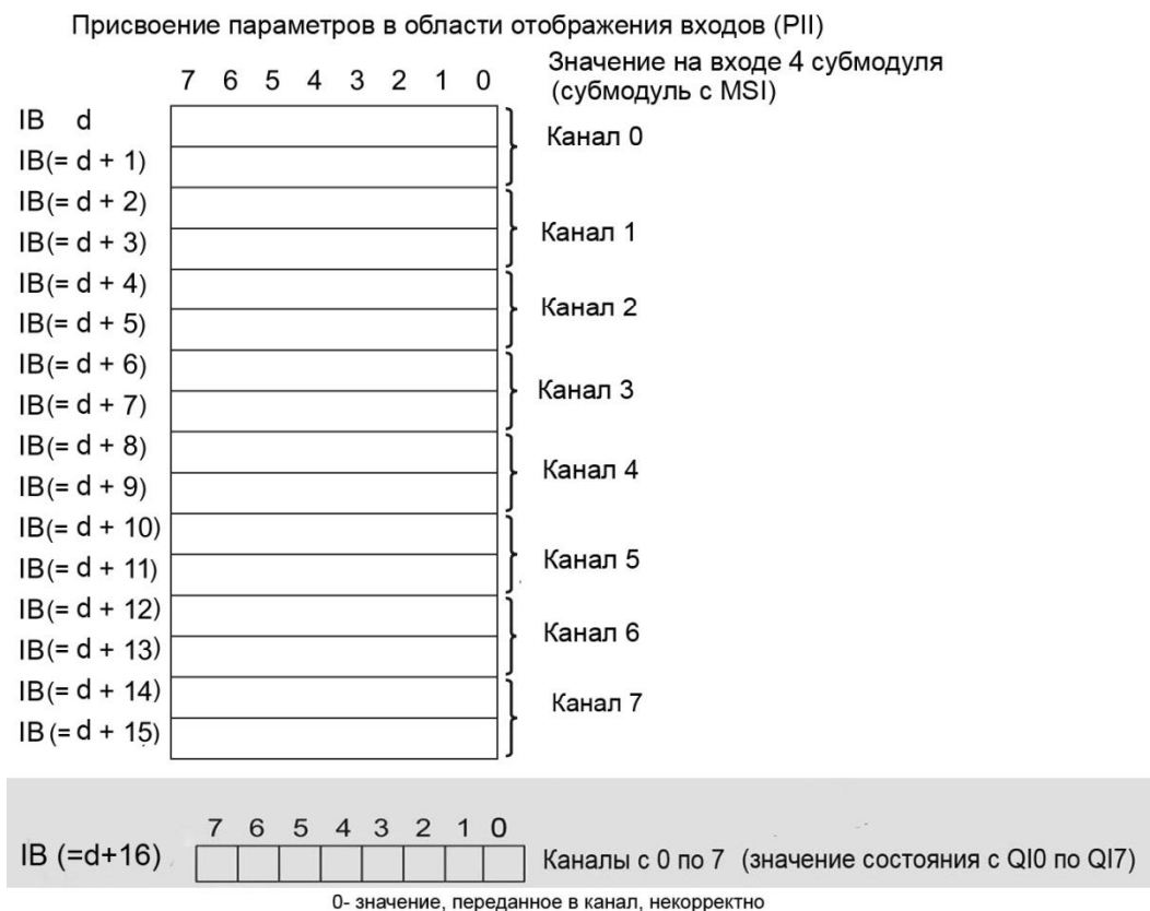
Рисунок 4-5 Адресное пространство для конфигурации 1 x 8 каналный AI 8xU/I HF MSI с оценкой состояния
