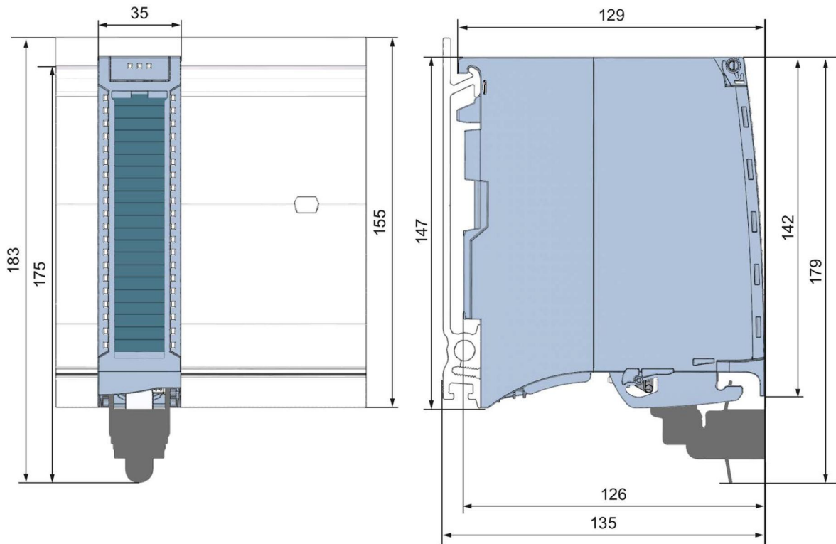
Рисунок А-1 Габаритный чертеж модуля AI 8xU/I HF
