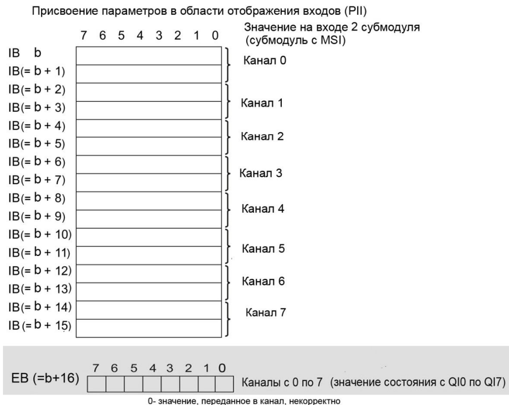
Рисунок 4-4 Адресное пространство для конфигурации 1x8 каналный AI 8xU/I HF MSI с оценкой состояния
